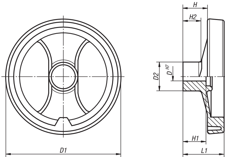
Passfedernut nach DIN 6885-1
